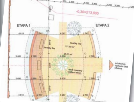
návrh kolumbária v západním rohu hřbitova
