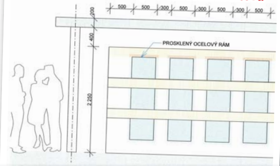
západní část kolumbária
